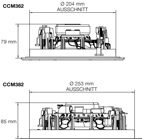
Abbildung 1 Öffnung und Einbautiefe
