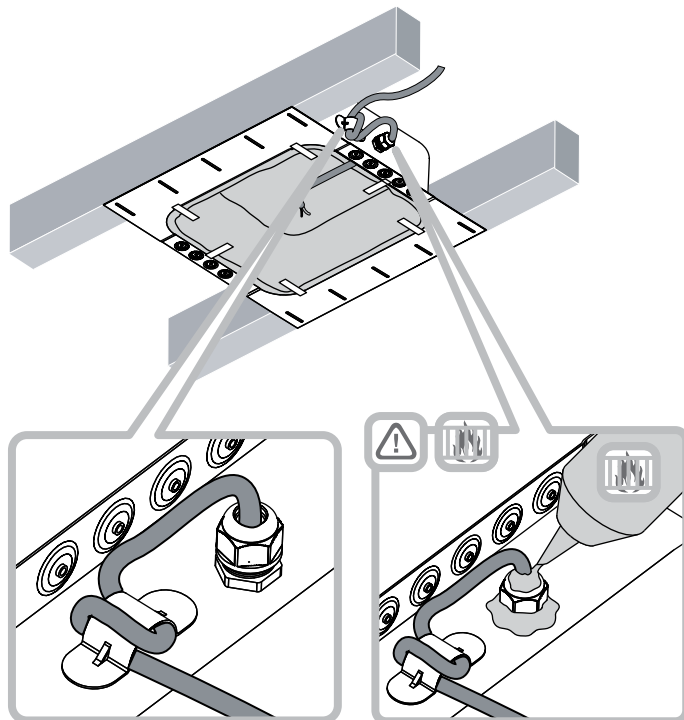
Afbeelding 11 Kabelbevestiging
