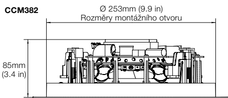
Obrázek 1 Montážní otvor a jeho rozměry
