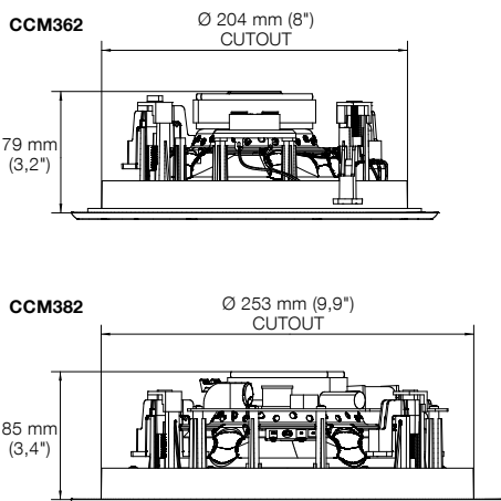
Afbeelding 1 Benodigde ruimte boven en achter
