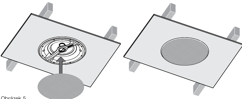
Obrázek 5 Přípevnění mřížky
