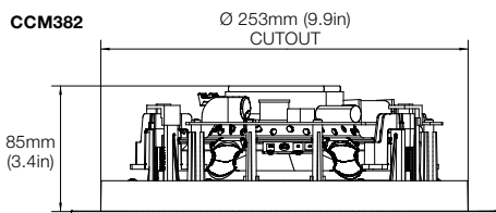
1. ábra Kivágási méretek
