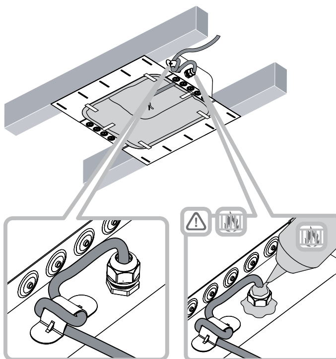
Abbildung 11 Installation des Kabels
