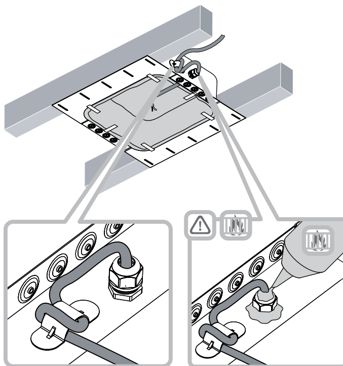
Obrázek 10 Připevnění Back-boxu k nosníkům
