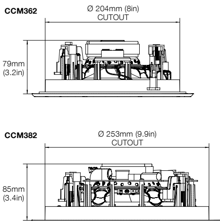
Diagrama 1 Espaço de abertura e profundidade necessários
